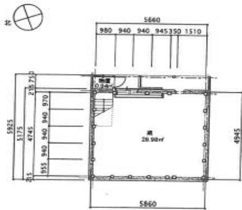
1階平面図 1/100 29.92㎡
